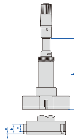
type C 50-200 mm, points de mesure en carbure de tungstène - trois points
