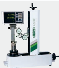
BANC DE PRÉRÉGLAGE D'OUTILS
