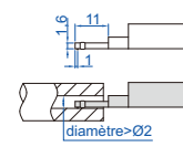
sonde à rainure profonde (en option), code ISR-C002-DGP1
