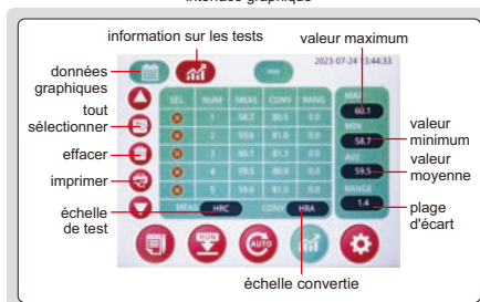
interface graphique
