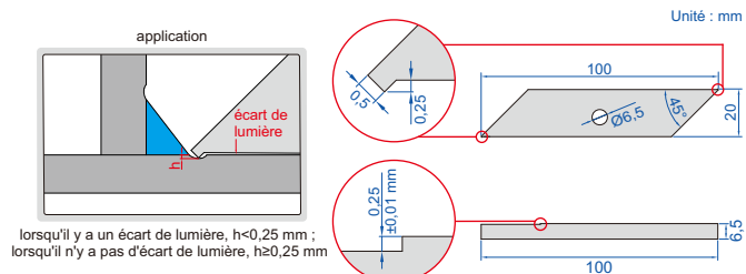
bloc d'étalonnage (inclus)
