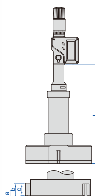
type C 50-150 mm, points de mesure en carbure de tungstène - trois points
