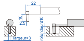
sonde à rainure profonde (en option), code ISR-C002-DGP1
