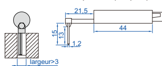
sonde à rainure profonde (en option), code ISR-C002-DGP1
